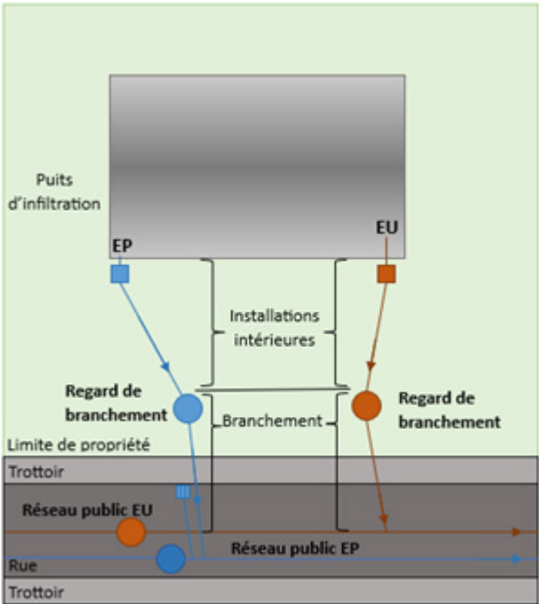
Réseau séparatif
