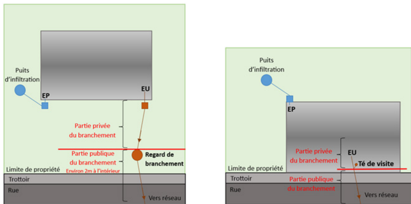
Limite privé-public
