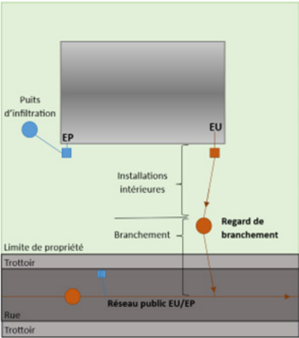
Réseau unitaire
