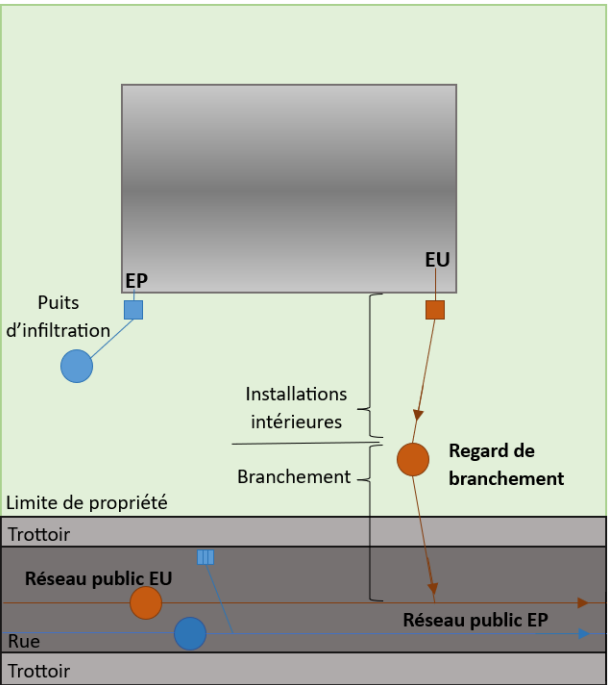
Réseau pseudo-séparatif
